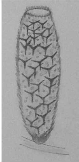
Leucosolenia
