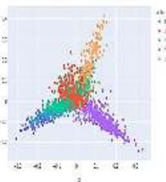
Clusterin
