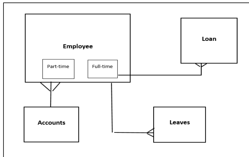
Figure 6: Example of EERD
