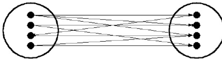
(d) Many-to-Many Mapping
